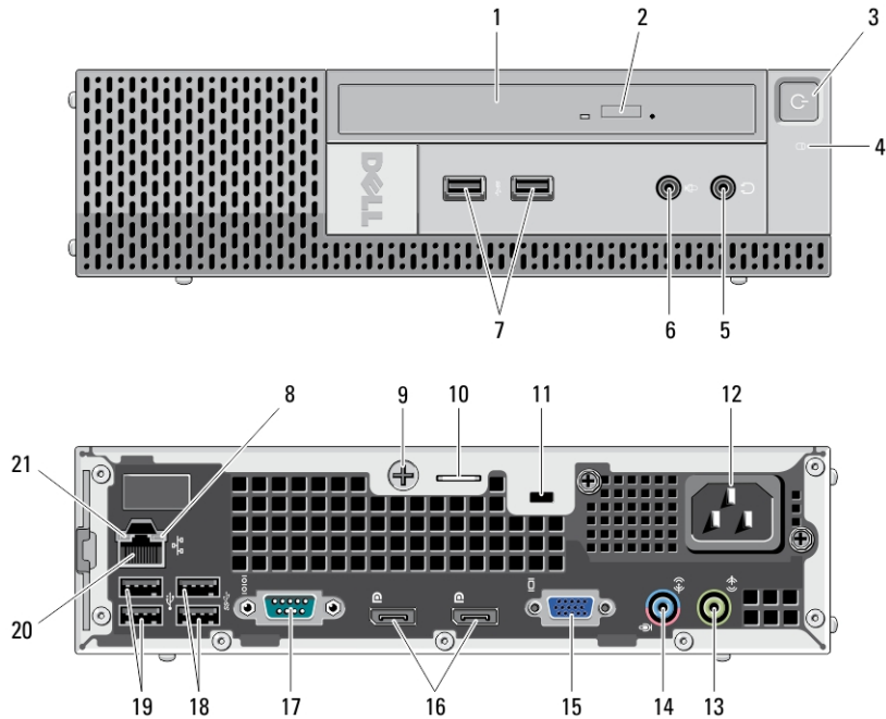
Afbeelding 5. Voor- en achteraanzicht — Ultra Small Form Factor
