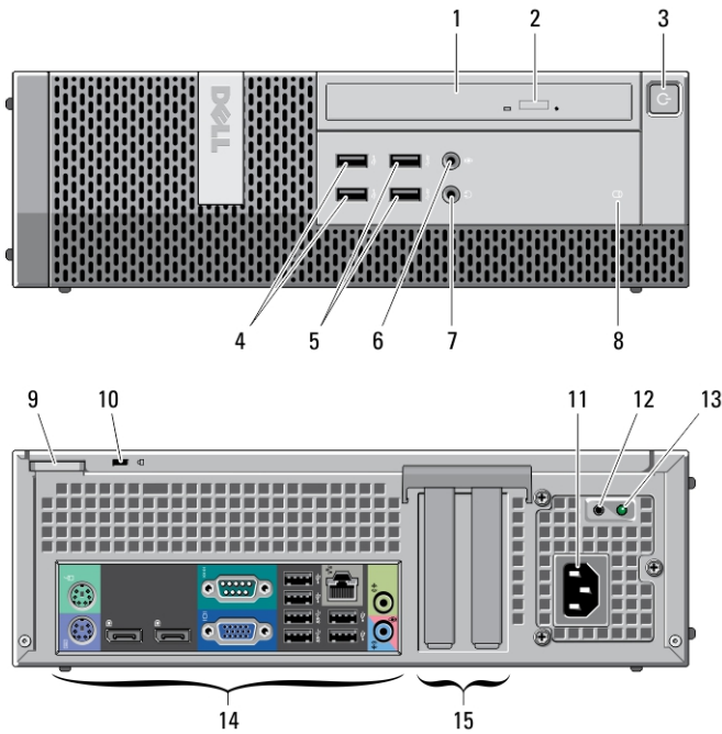
Afbeelding 3. Aanzicht achterpaneel van Small Form Factor
